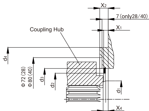
Splined shaft DIN (spline according to DIN 5480)
